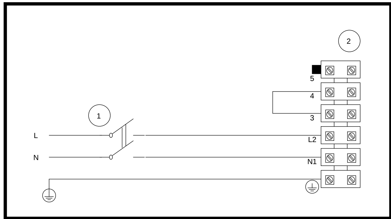
FACTORY SETTING SCHEME - SCHEMA IMPOSTAZIONE DI FABBRICA WIRING FOR VMAX ONLY - COLLEGAMENTO PER FUNZIONAMENTO CONTINUO ALLA VMAX
