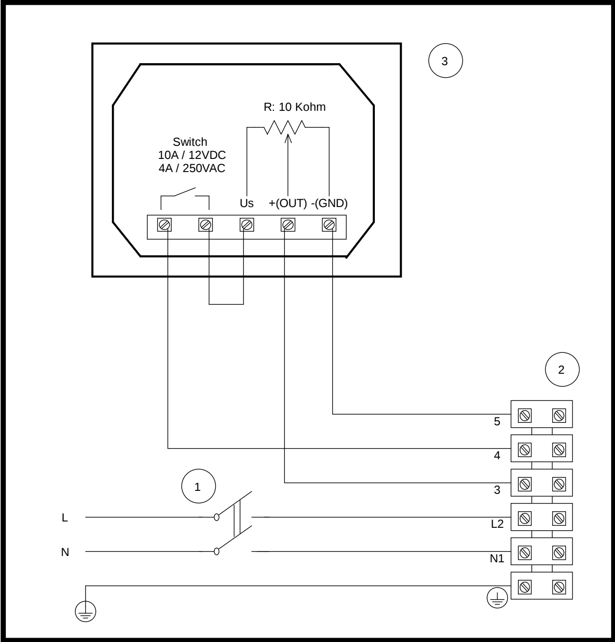
WIRING TO CONTROL BOX code 12828 - COLLEGAMENTO A SCATOLA COMANDI codice 12828
