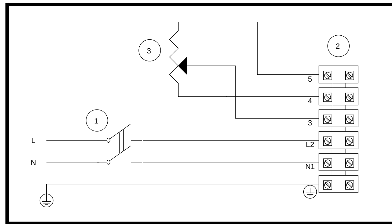
WIRING TO STANDARD TRIMMER - COLLEGAMENTO A POTENZIOMETRO STANDARD
