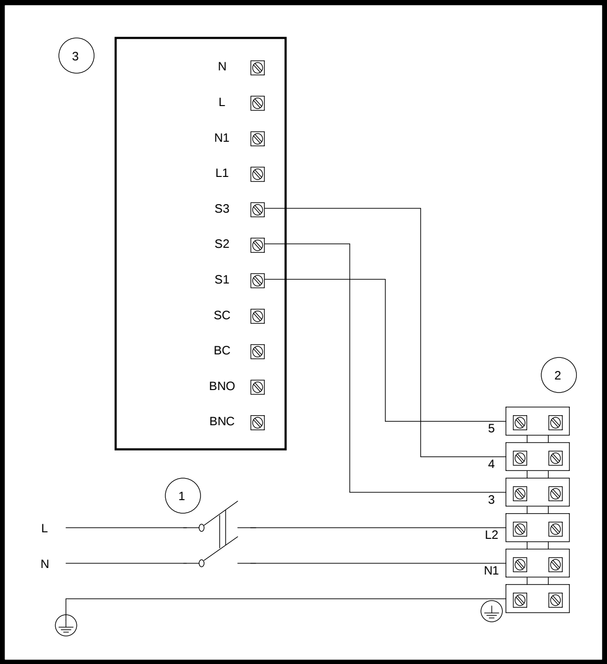
WIRING TO CONTROL BOX code 12832 - COLLEGAMENTO A SCATOLA COMANDI codice 12832
